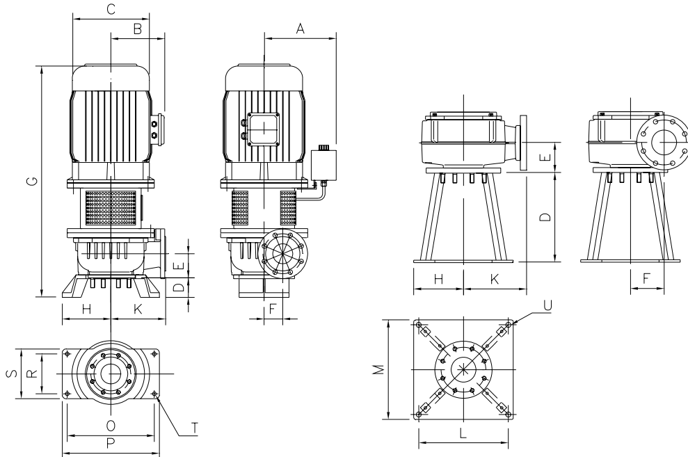
BW4030-VS/BW4040-VS/BW4041-VS
