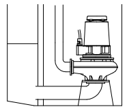
A Überflutbare Trockenaufstellung: vertikal und horizontal mit Kühlsystem und Grundplatte. Druckstutzen: 150mm Saugstutzen: 200mm
