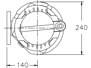
V Onderwaterkoppeling: Type V50
