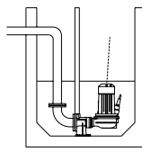
V Onderwaterkoppeling: Type V50
