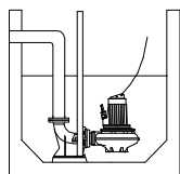
V Onderwaterkoppeling: Type V100
