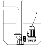
V Guide bar coupling: Type V65-N
